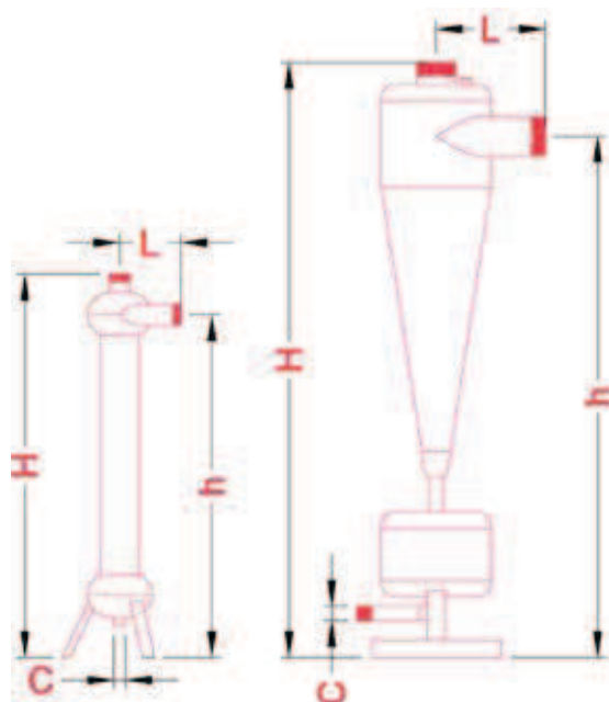
Filtro Serie "HCY" Modular 2"
